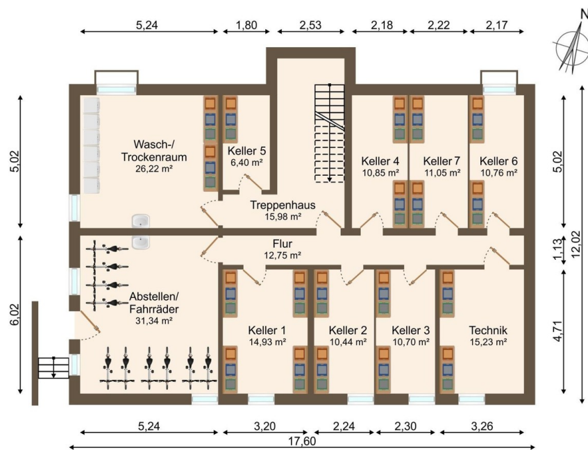
Grundriss Keller 2
