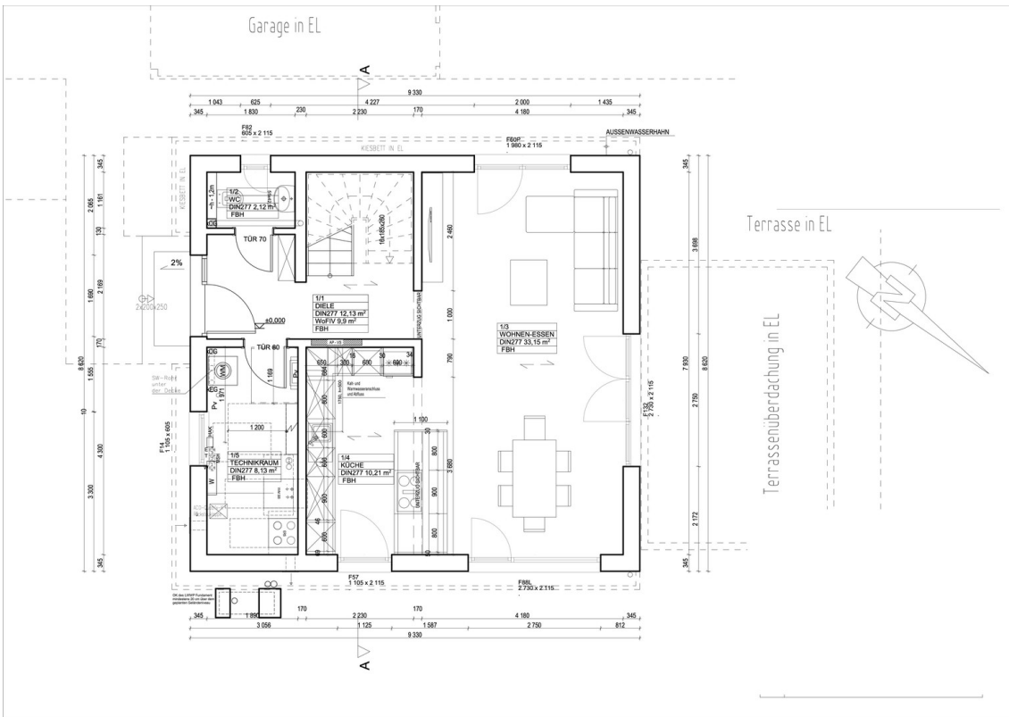
Grundriss EG
