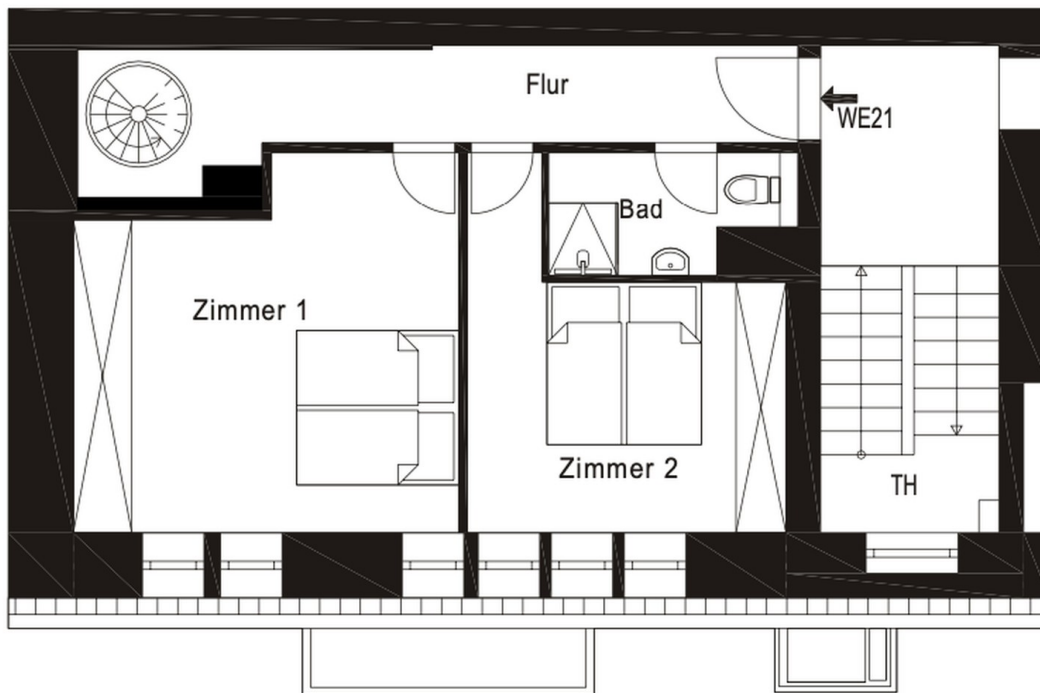
Grundriss DG
