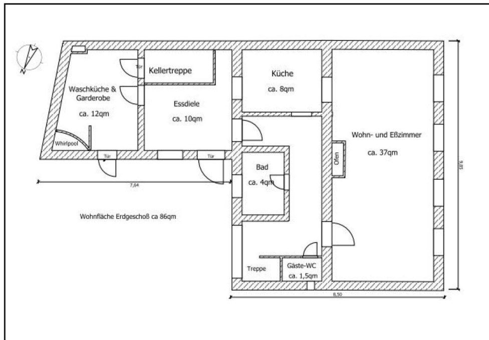
Grundriss EG.
