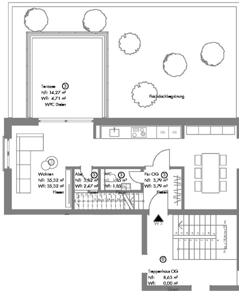
Wohnung 3 OG
