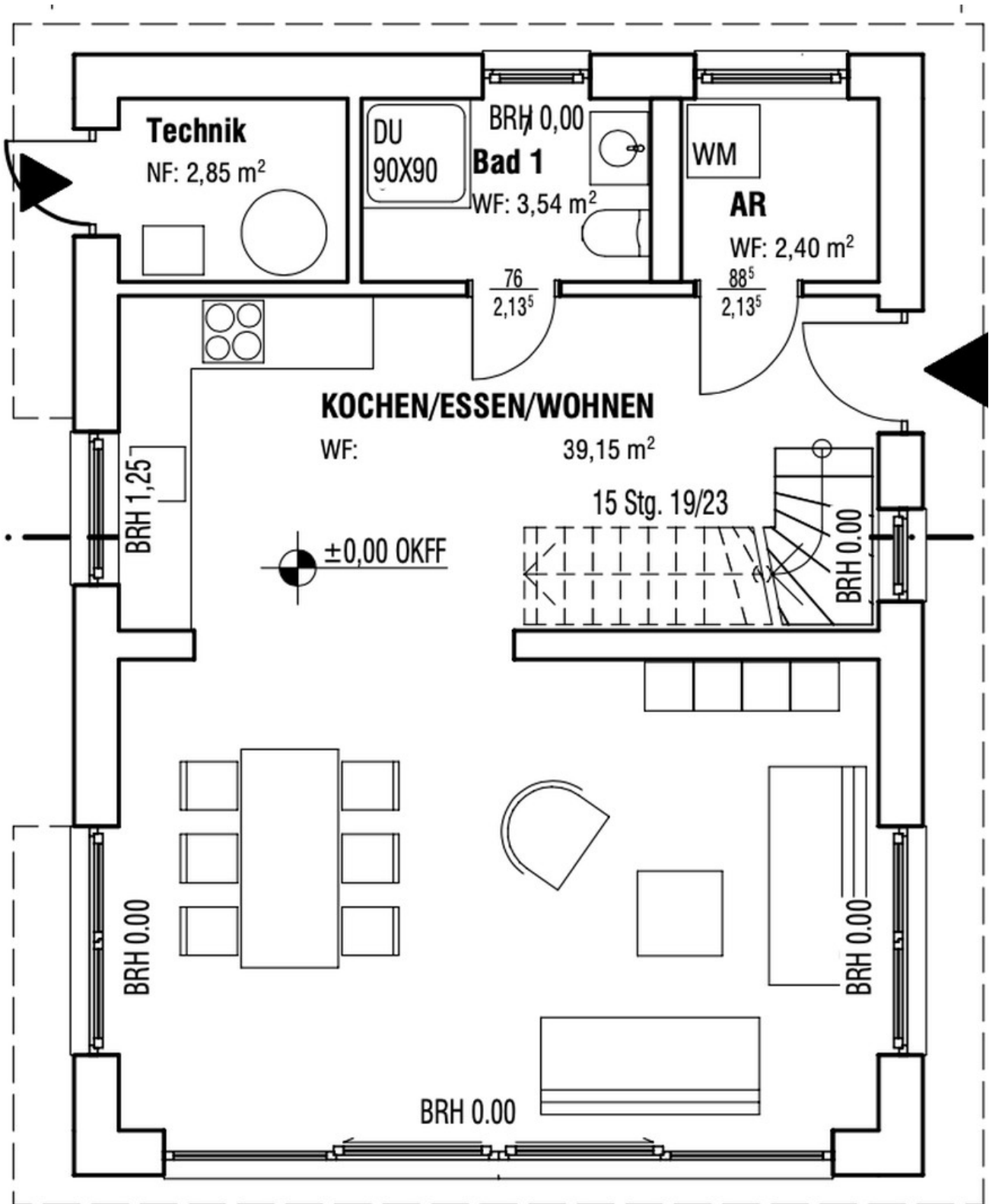
Erdgeschoss
