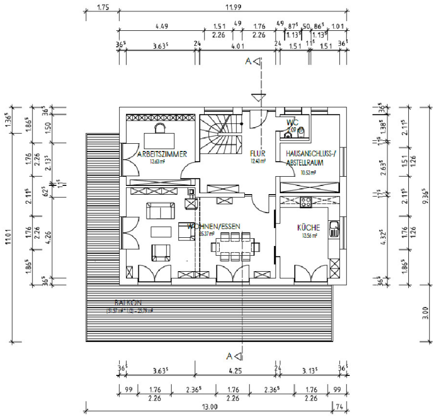
GRUNDRISS ERDGESCHOSS
