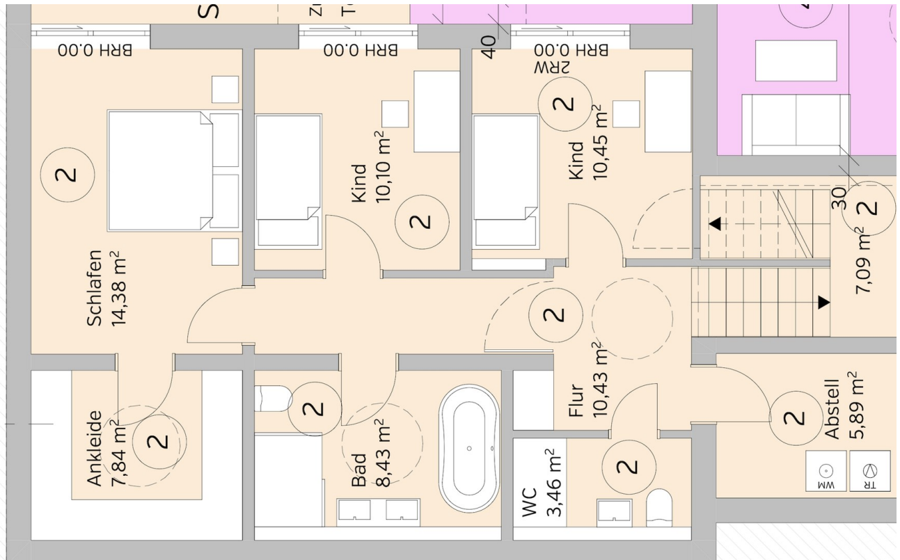
Grundriss Schlafenebene
