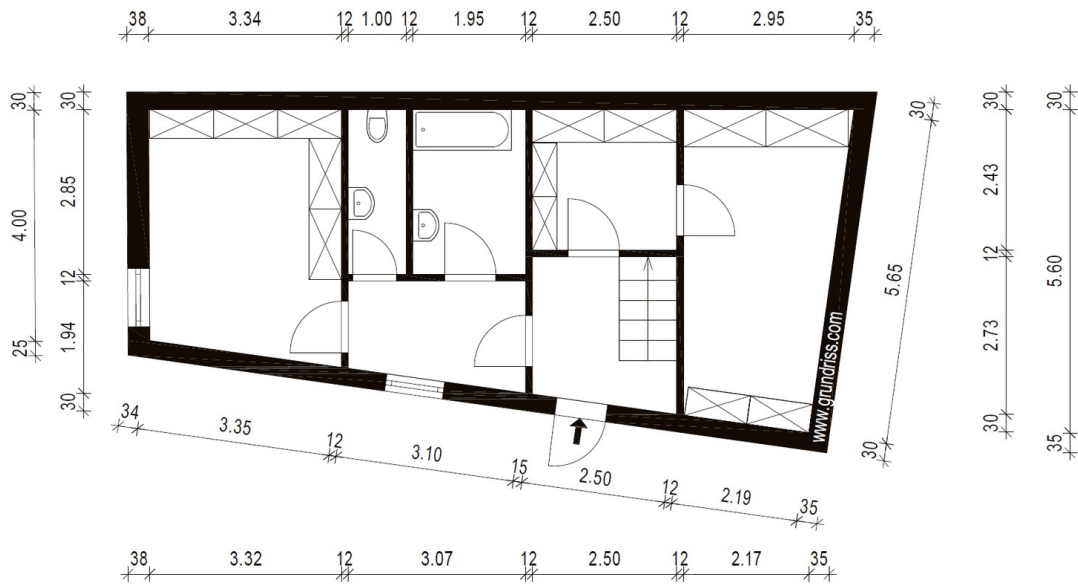
Erdgeschoss
