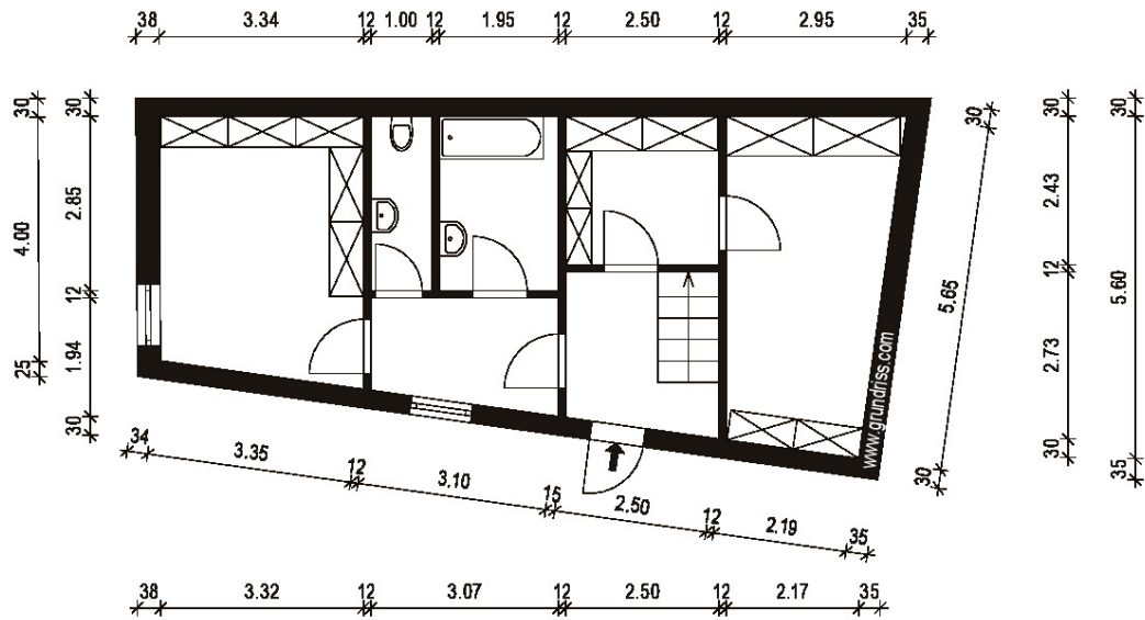
Erdgeschoss
