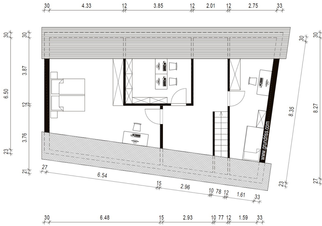
Dachgeschoss
