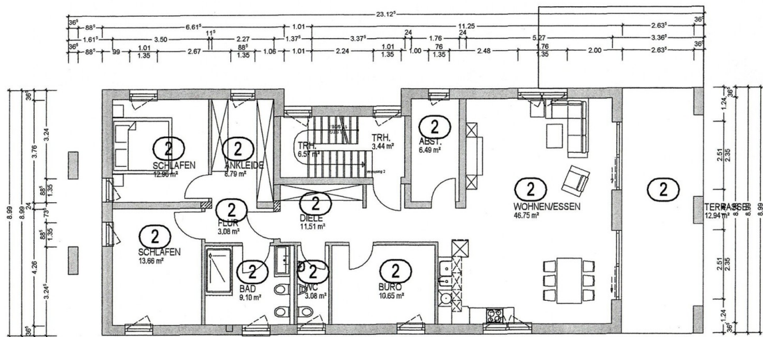
121 - 1. OBERGESCHOSS
