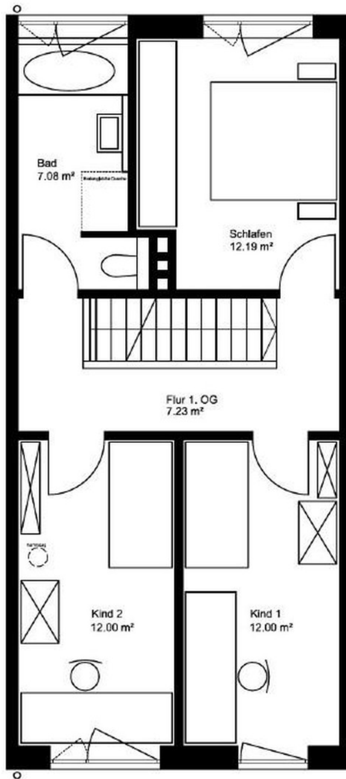
1. OG
