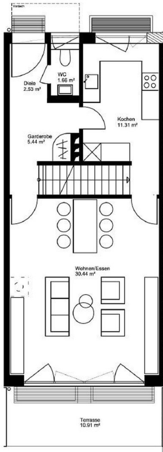
Erdgeschoss
