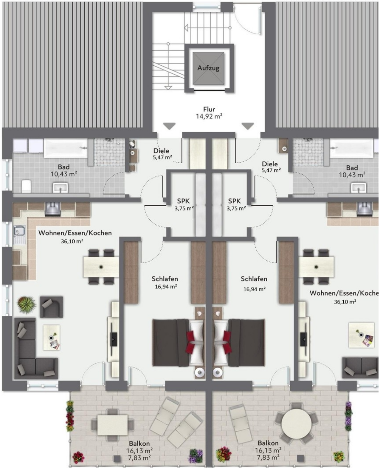
Grundriss_Obergeschoss
