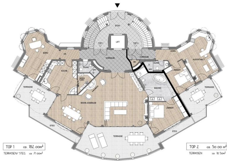
GRUNDRISS ERDGESCHOSS HAUPTGEBÄUDE
