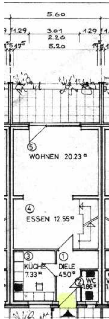
Erdgeschoss
