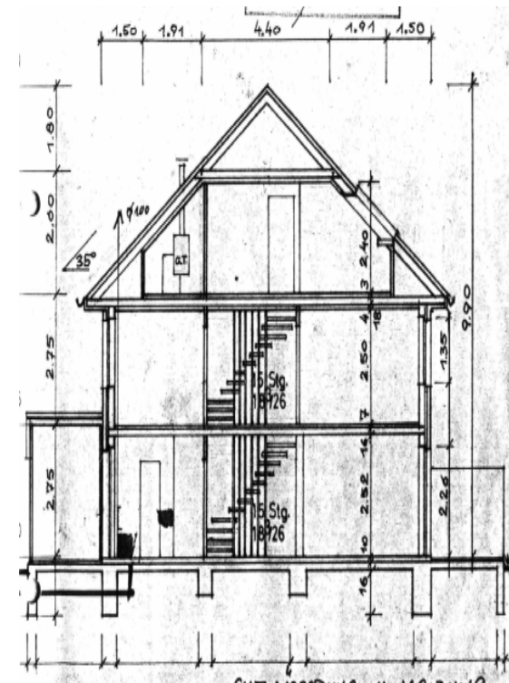
Querschnitt
