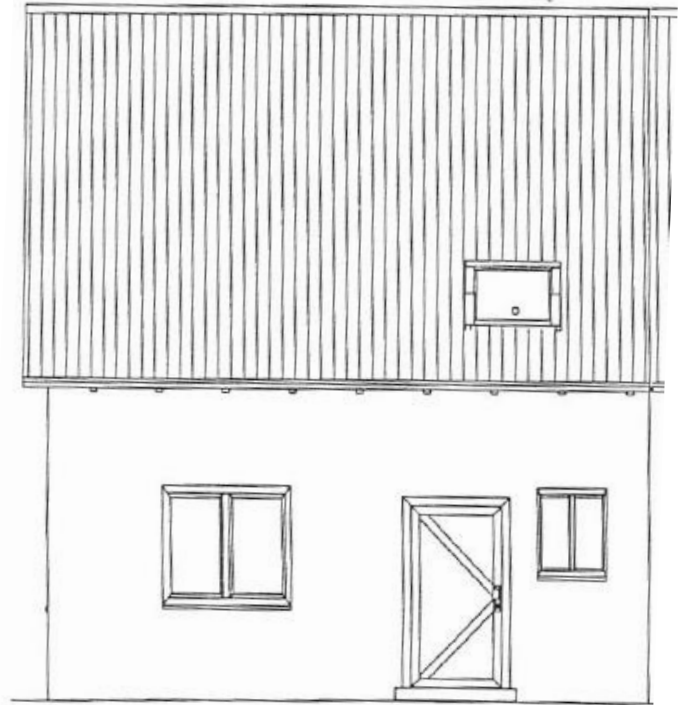
Nordansicht
