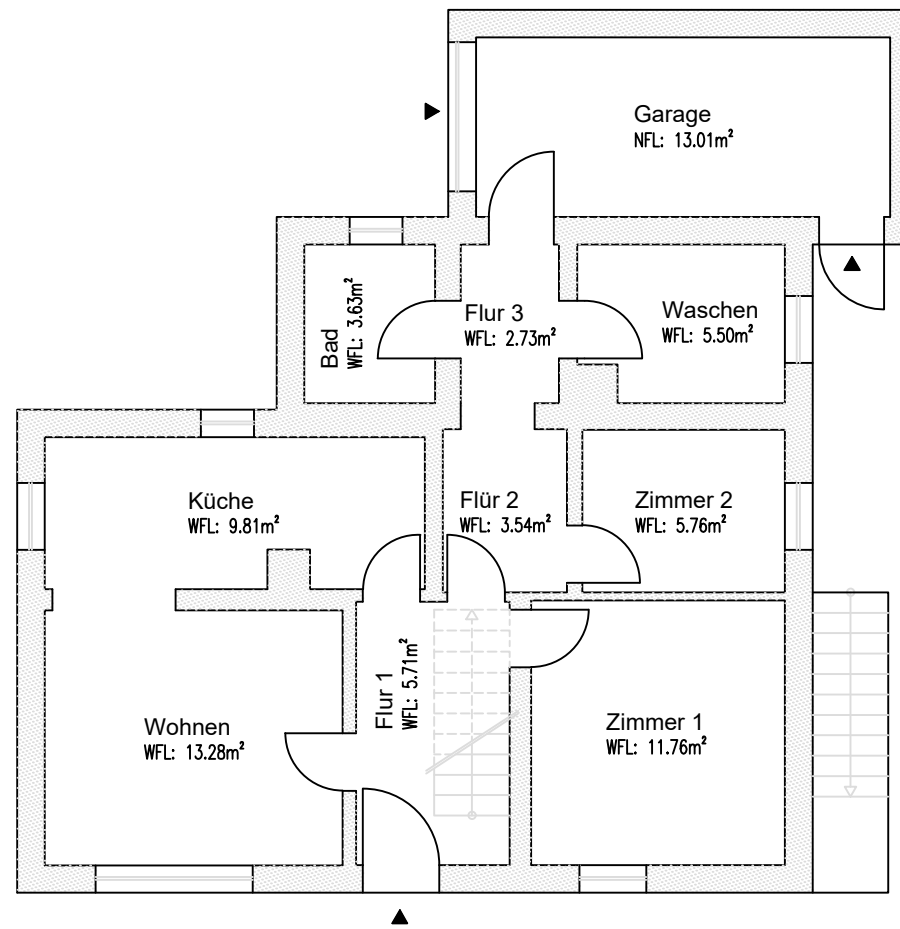
ERDGESCHOSS
