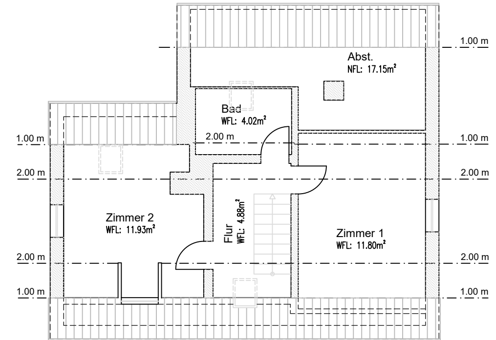
DACHGESCHOSS
