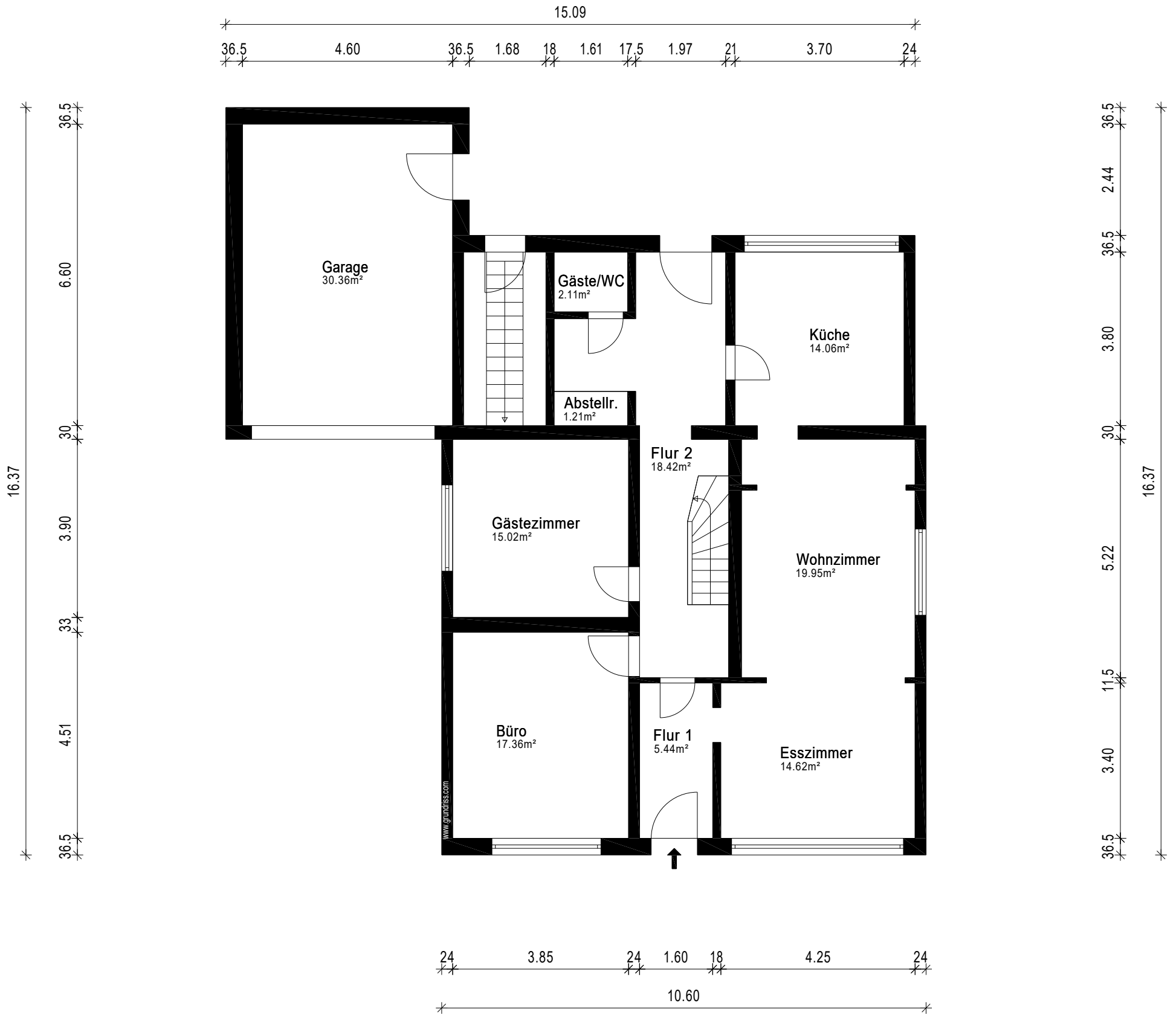
Erdgeschoss
