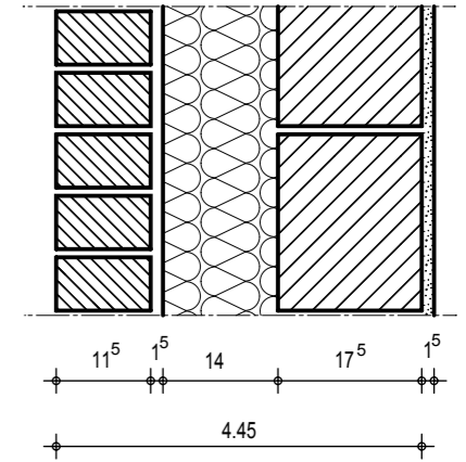
Außenwand (Haus) M1:10
