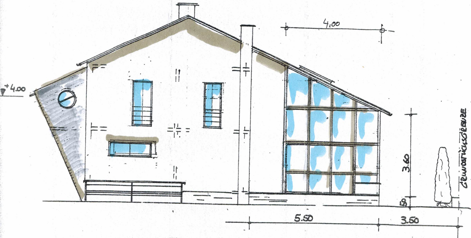
Ansicht West
