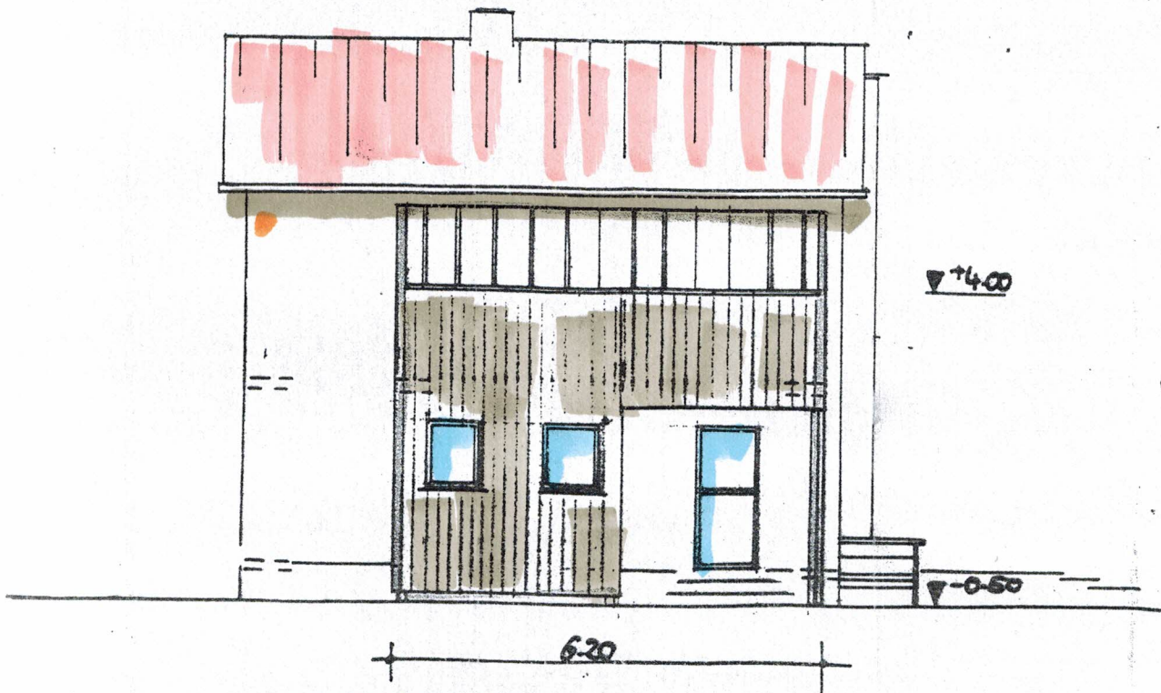
Ansicht Nord
