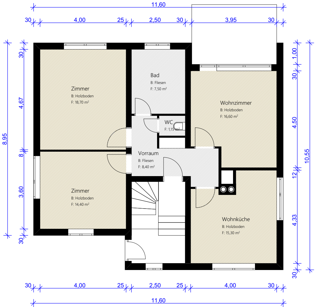
Grundriss Erdgeschoß
