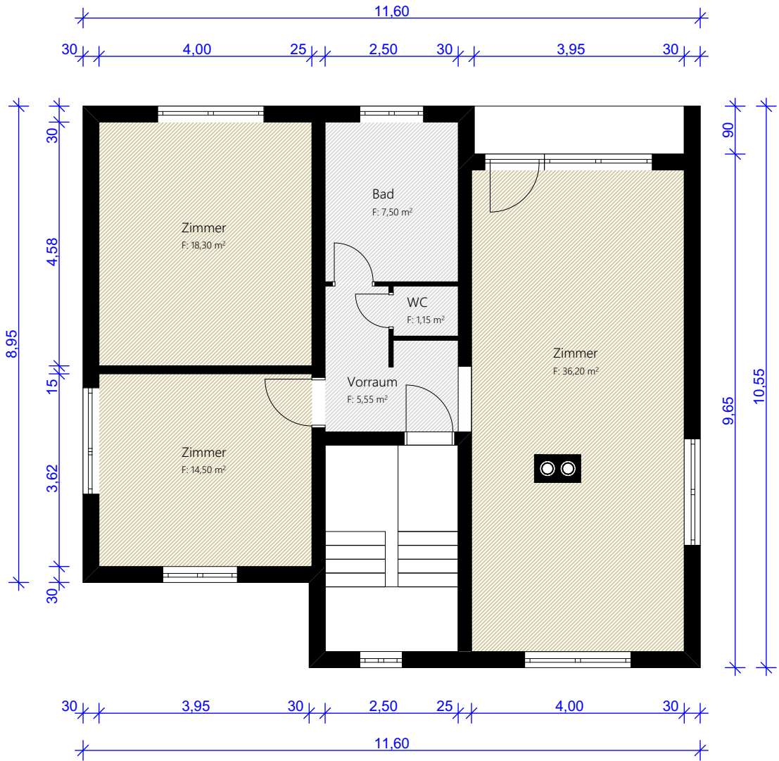
Grundriss Obergeschoß
